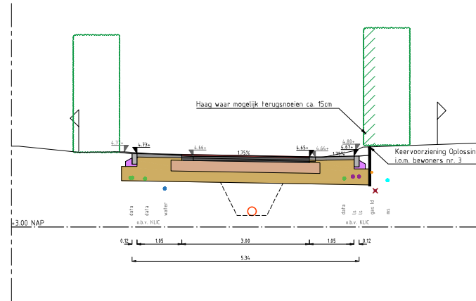
Doorsnede G-G Schaal 150
