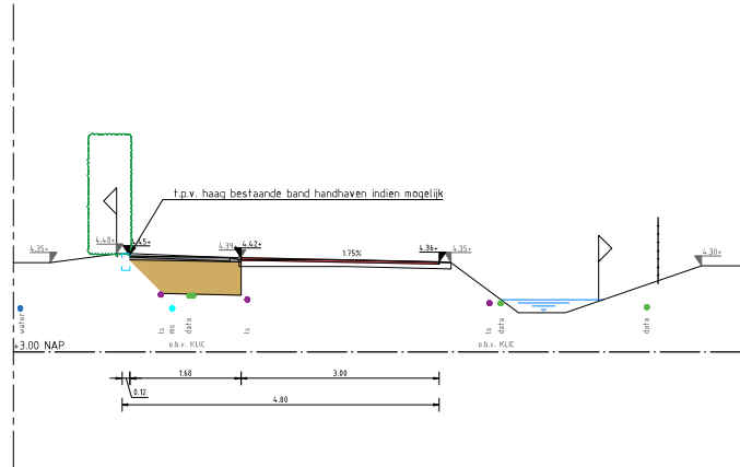
Doorsnede J-J Schaal 150
