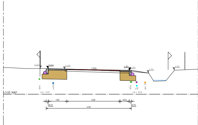
Doorsnede I-I Schaal 150
