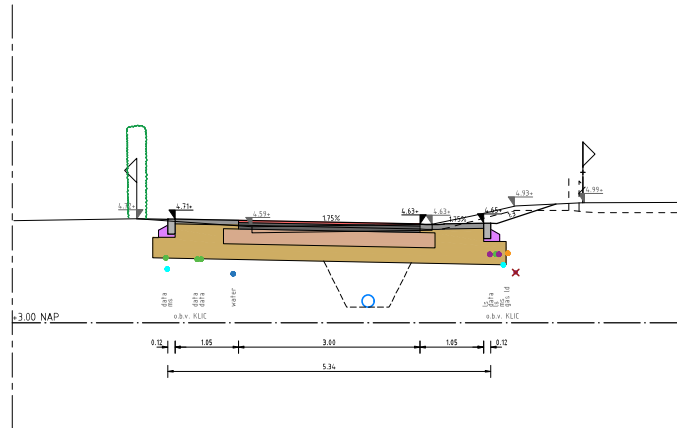
Doorsnede F-F Schaal 150
