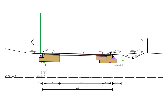
Doorsnede H-H Schaal 150
