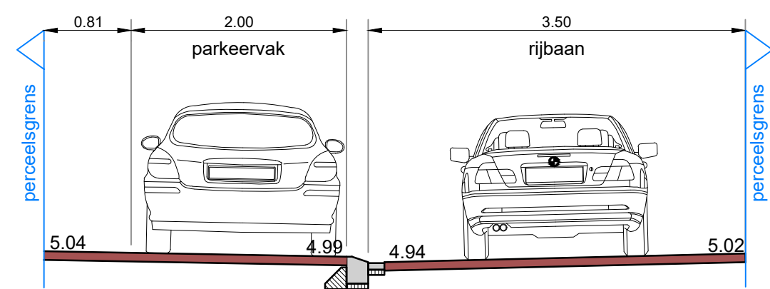
dwarsprofiel A-A schaal: 1 : 50
