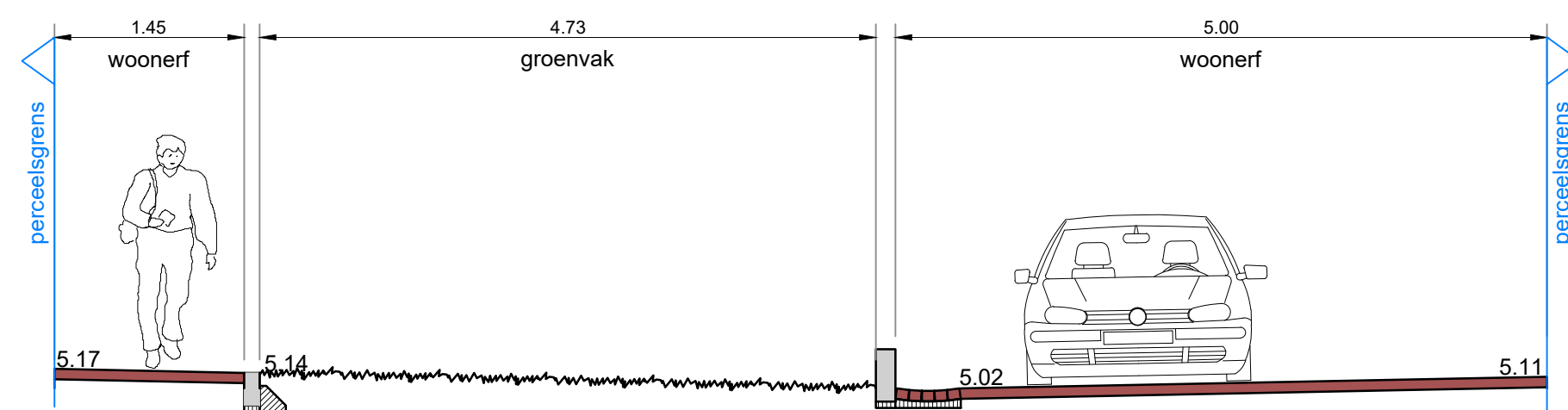
dwarsprofiel B-B schaal: 1 : 50
