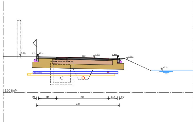
Doorsnede A-A Schaal 150
