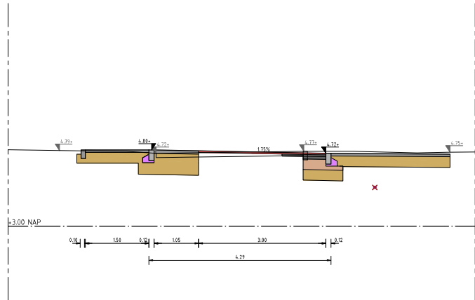
Doorsnede E-E Schaal 150
