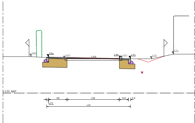
Doorsnede C-C Schaal 150
