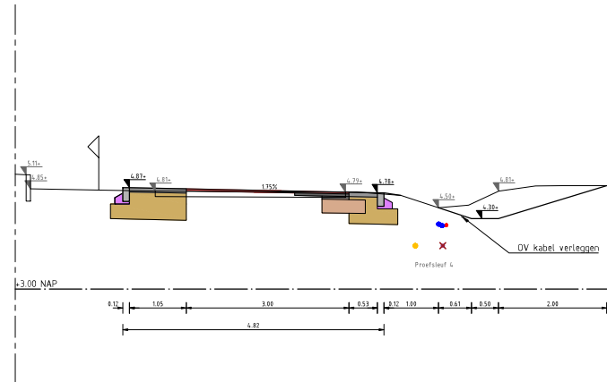
Doorsnede D-D Schaal 150
