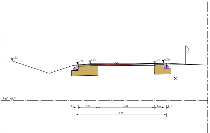
Doorsnede B-B Schaal 150
