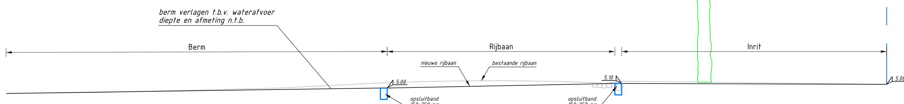
Dwarsprofiel A-A schaal 1:50
